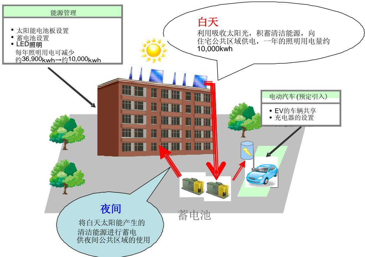
CREVIA 二子玉川有效利用太阳能电池板、定置用蓄电池系统的示意图
