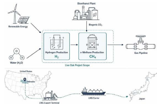
Live Oak プロジェクトにおける e-メタン製造と日本への輸出スキーム
